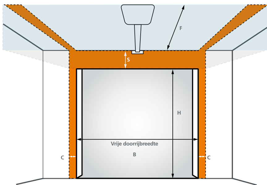
B = breedte, H = hoogte, C = zijruimte, S = bovenruimte, F = diepte
