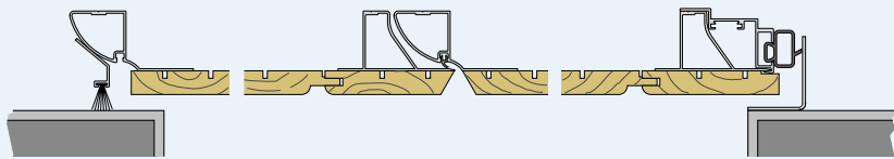
Aluminium frameconstructie
